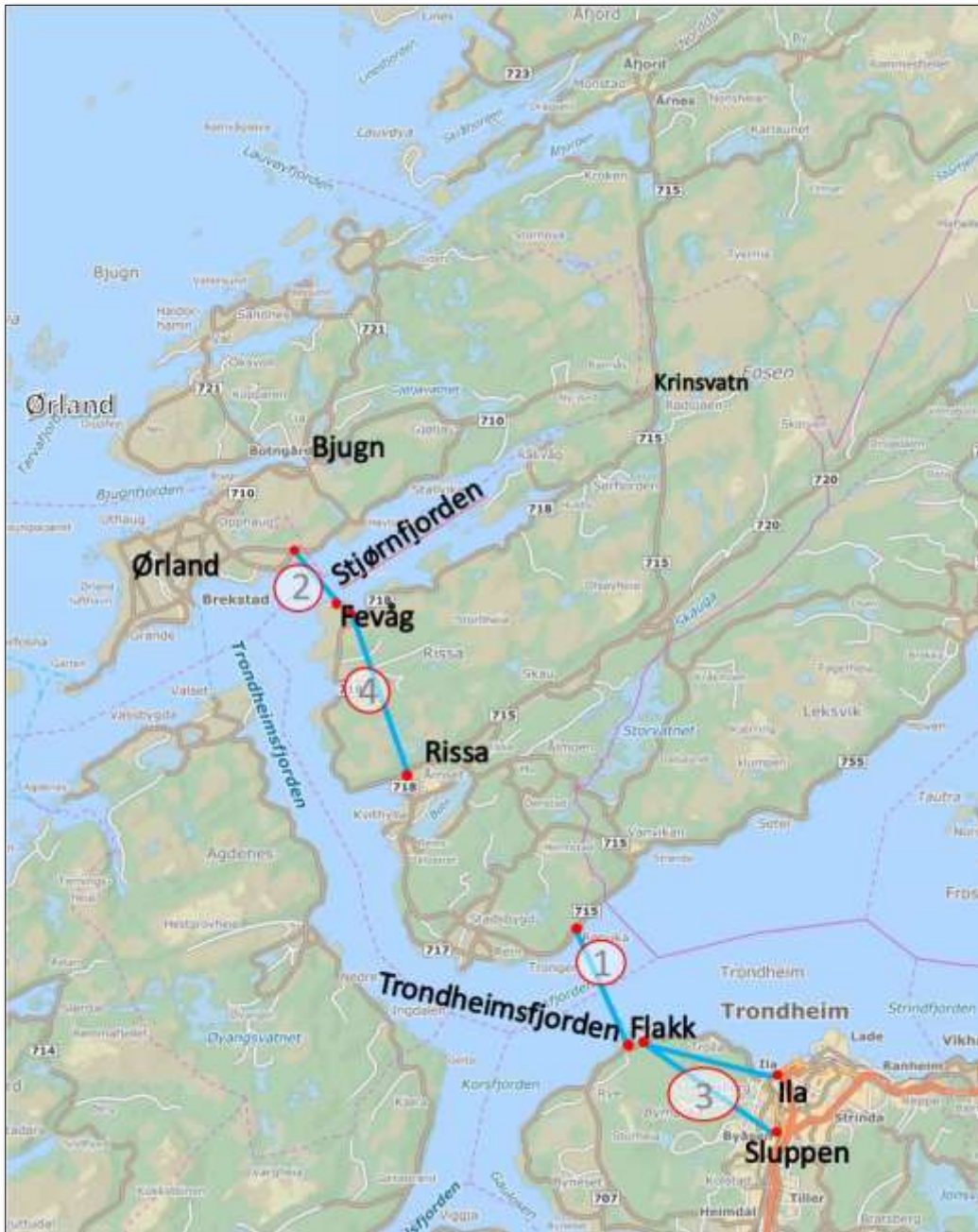
Figur 2 - Vegtiltakene i analysen, grovt skissert, nummerert etter utbyggingsrekkefølgen som er forutsatt
