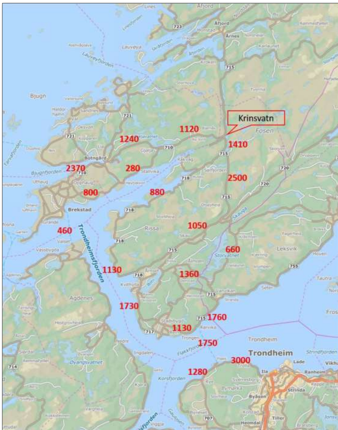
Figur 5 – Dagens vegnett, markeringene er ÅDT fra 2015 (Kilde: Statens vegvesen)
